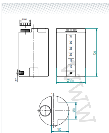
GEL.TANK PE - 35l
