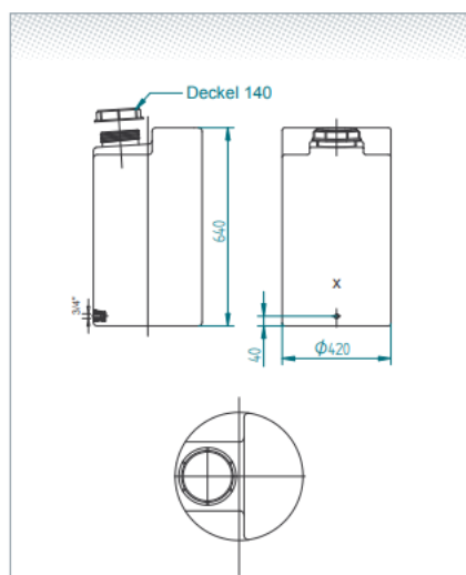
GEL.TANK PE - 60l
