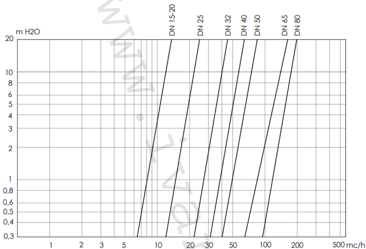
Tabulka Kv - DN
