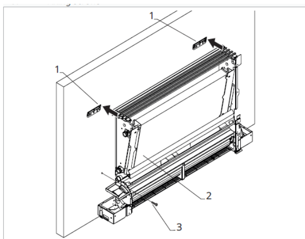
1 = montážní držáky 2 = Jednotka fancoilu 3 = upevňovací šroubky
