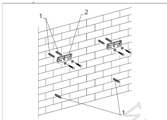
1 = hmoždinky 2 = montážní držáky
