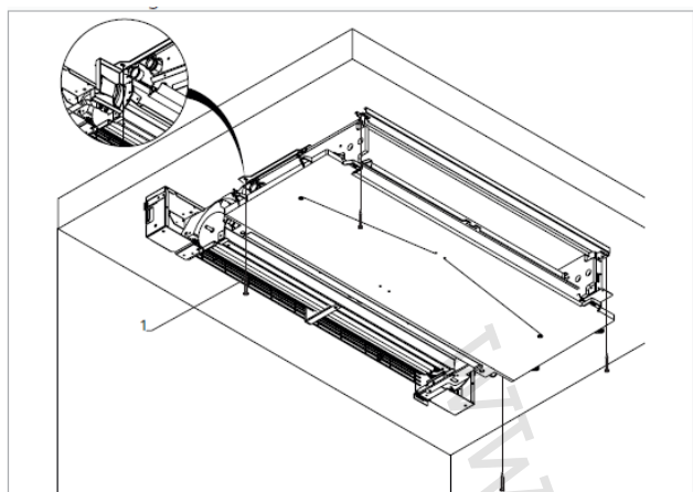
1 = Upevňovací šroubky
