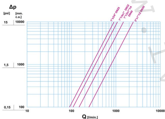
GRAF TLAKOVÝCH ZTRÁT
