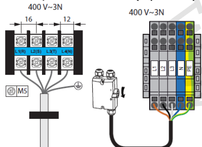
VNITŘNÍ JEDNOTKA
