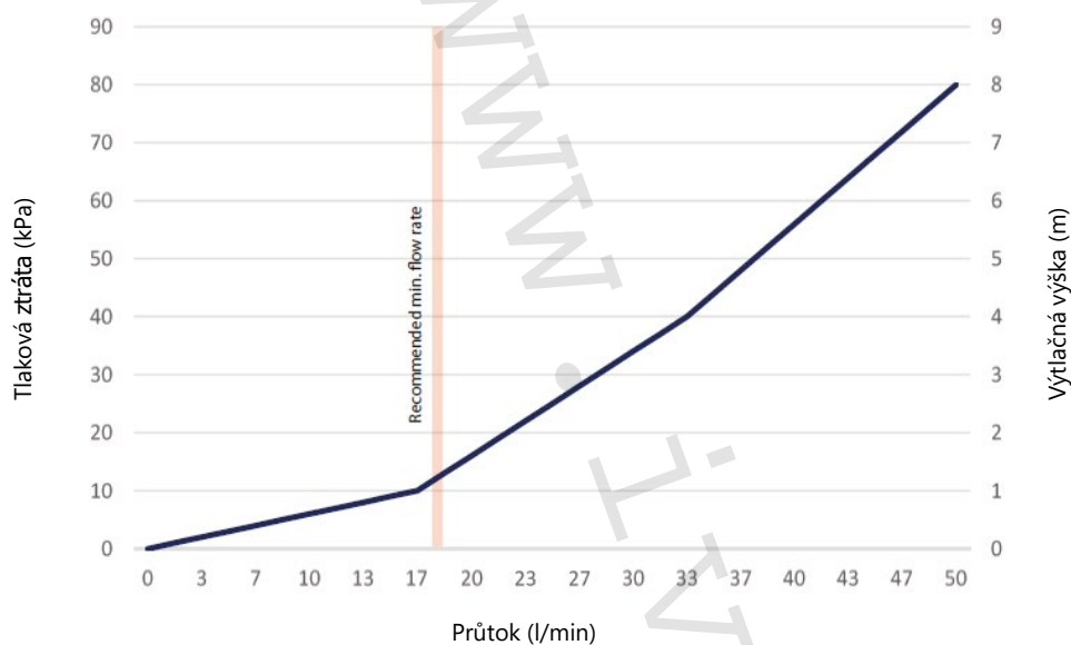
Vnitřní tlaková ztráta samostatné venkovní jednotky Athena
