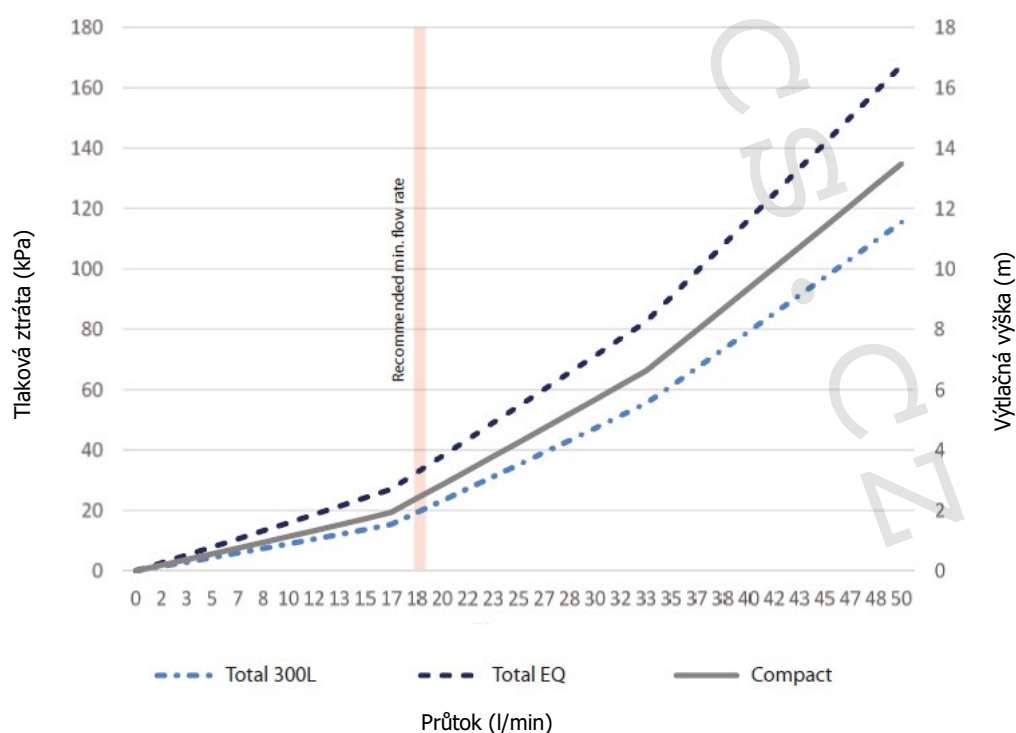
Celková tlaková ztráta vnitřní + venkovní jednotky
